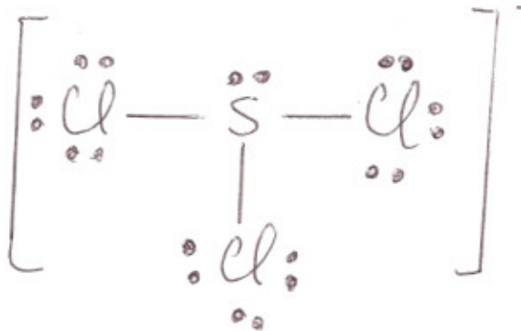
h) \text{SCl}_3^+ ion
