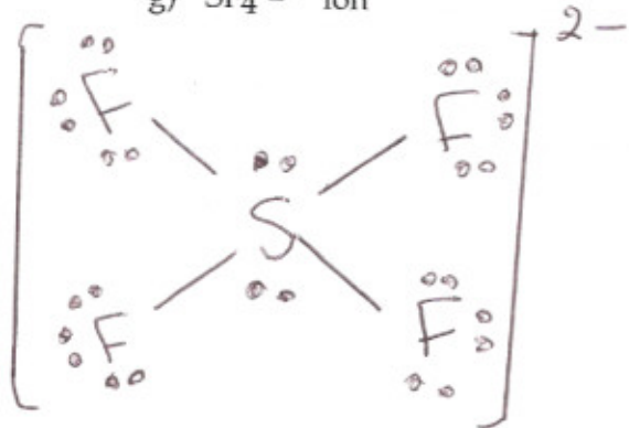
g) \text{SF}_4^{2-} ion
